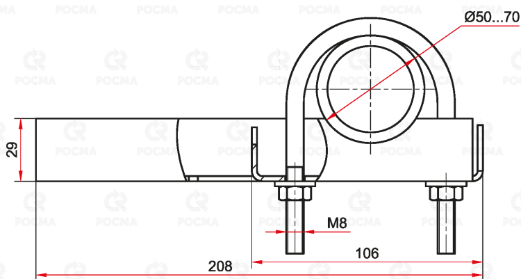
Кронштейн на трубу для ТМД-2
